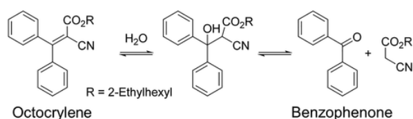
Figure 1 - Transformation de l'octocrylène en benzophénone
