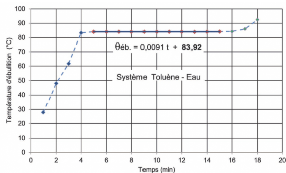
Figure 2 - Étude de l'hétéroazéotrope toluène-eau - Relevé expérimental de température en tête de colonne au cours du temps permettant la détermination de la température de l'hétéroazéotrope .
