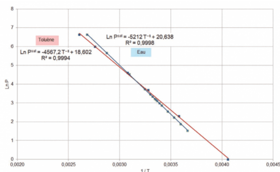
Figure 3 - Étude théorique de l'hétéroazéotrope toluène-eau (calcul et tables)
