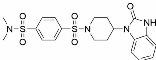
Figure 1 - Structure du composé NM102, qui présente des propriétés antimicrobiennes
