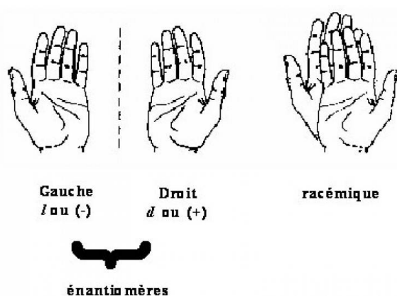
Figure 2 - Illustration de la notion de chiralité
