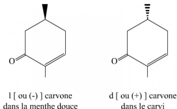
Figure 3 - Les deux énantiomères de la carvone
