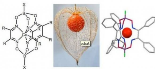
Figure 1 - Cobalt en cage
