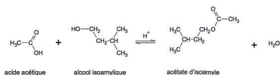
Figure 1 - Equation de la synthèse de l'acétate d'isoamyle
