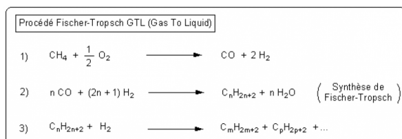
Figure 2 - Le procédé Fischer-Tropsch
