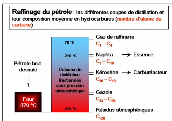
Figure 1 - Le raffinage du pétrole
