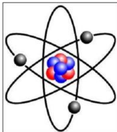
Figure 3. Modèle planétaire
