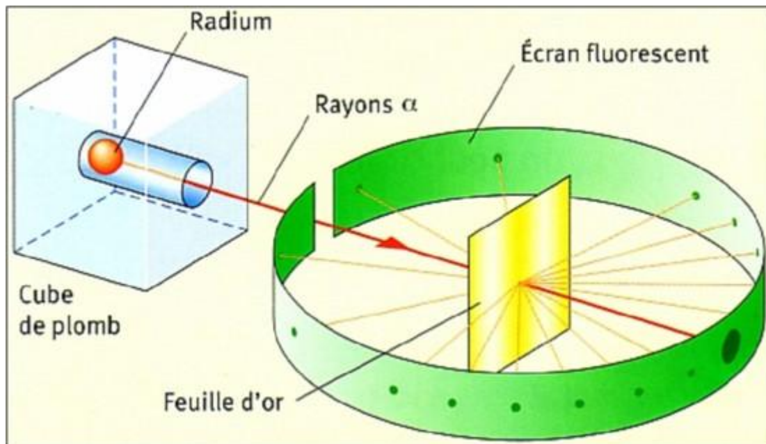
Figure 2. Expérience de Rutherford
