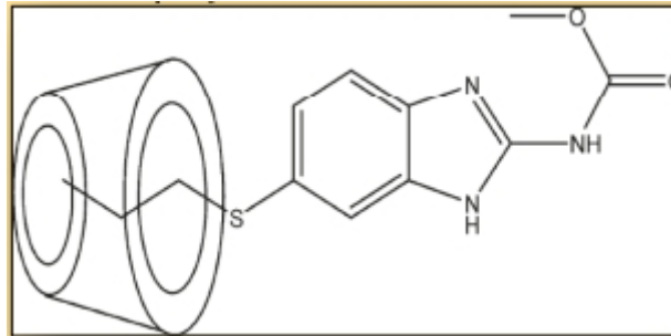
Figure 4. Agent anti-cancer ABZ complexé à une bêta-cyclodextrine.
