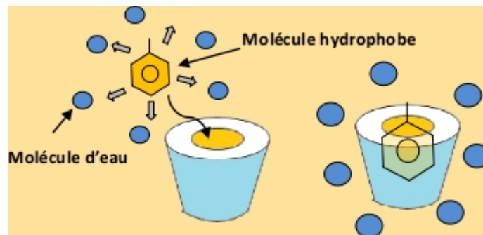
Figure 2. Cavité d'une cyclodextrine - effet d'encapsulation.
